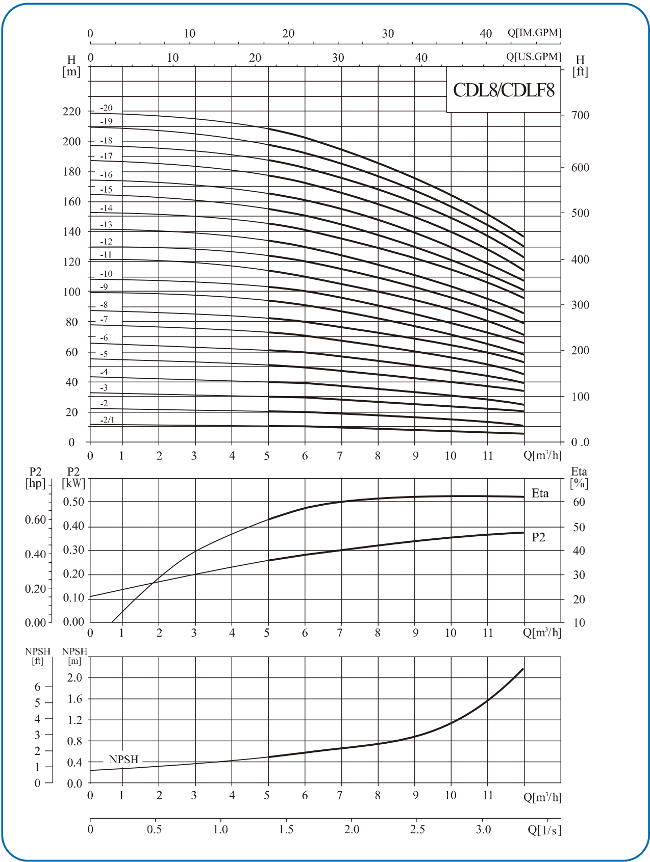
性能曲线
