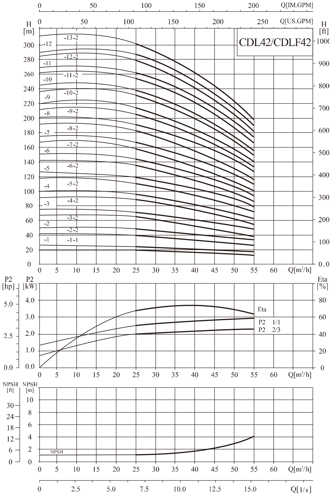
性能曲线
