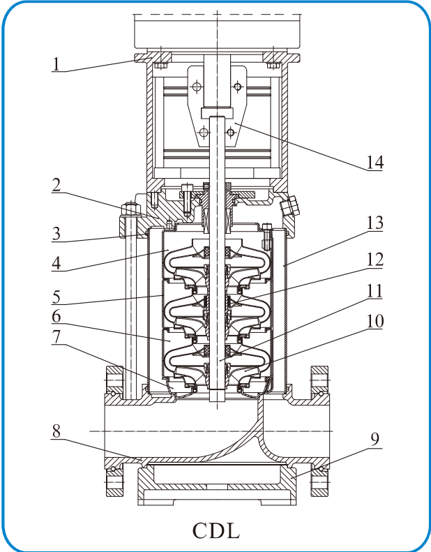
截面图 CDL,CDLF32,42,65,85
