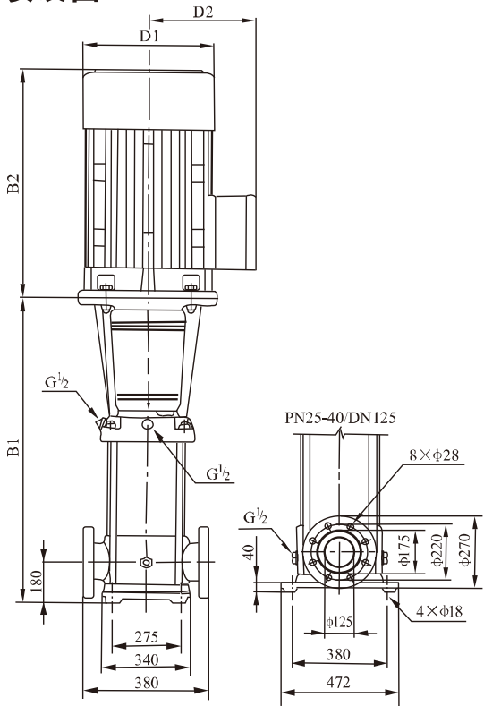
安装图
