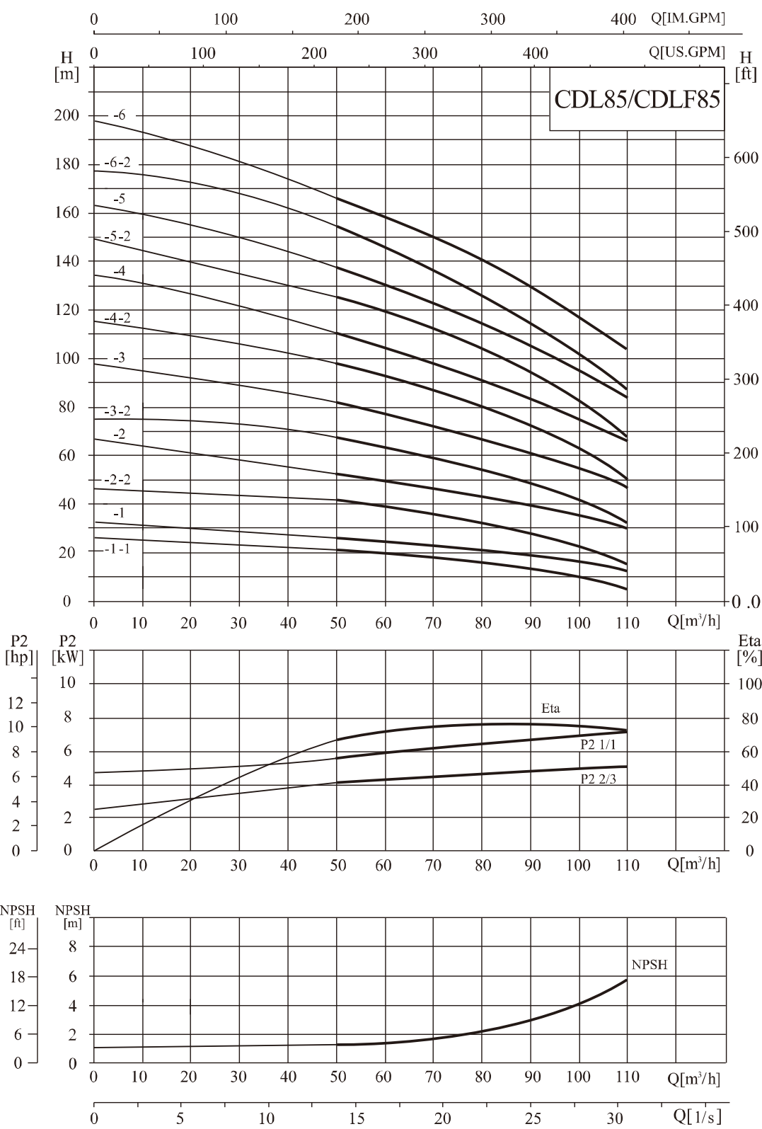
性能曲线
