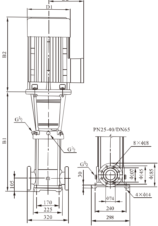
安装图
