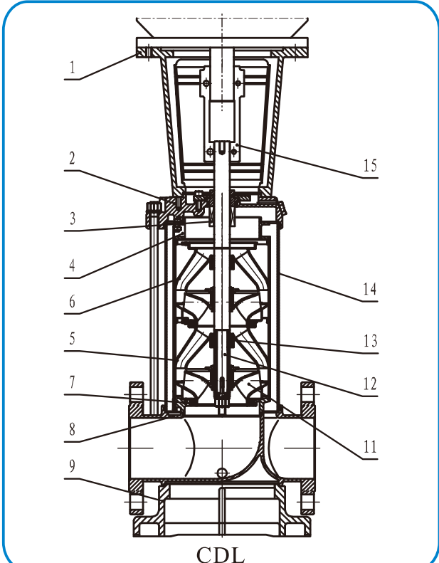
截面图 CDL,CDLF120,150,200
