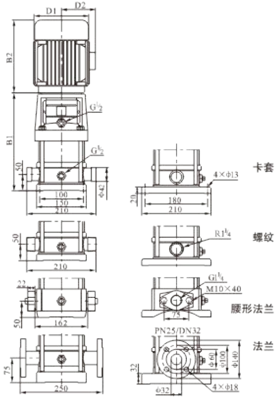
安装图
