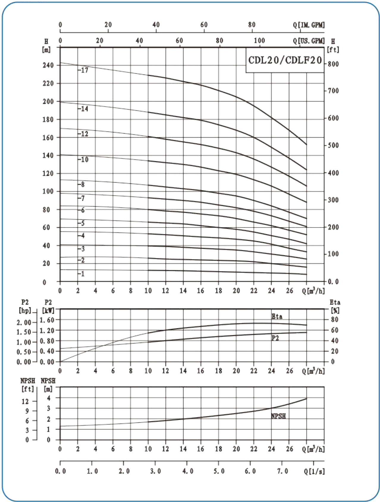
性能曲线
