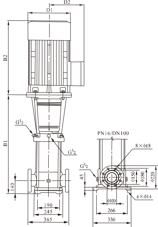
安装图
