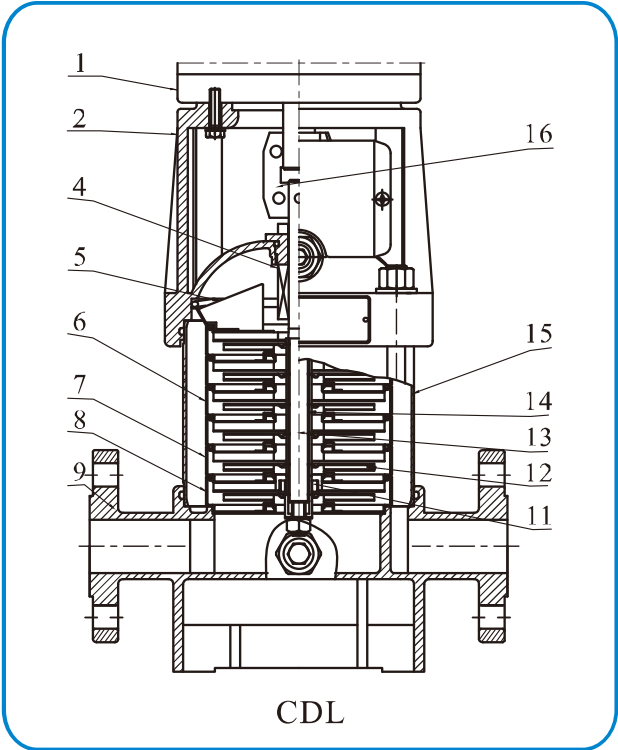
截面图CDL,CDLF1,2,3,4,5
