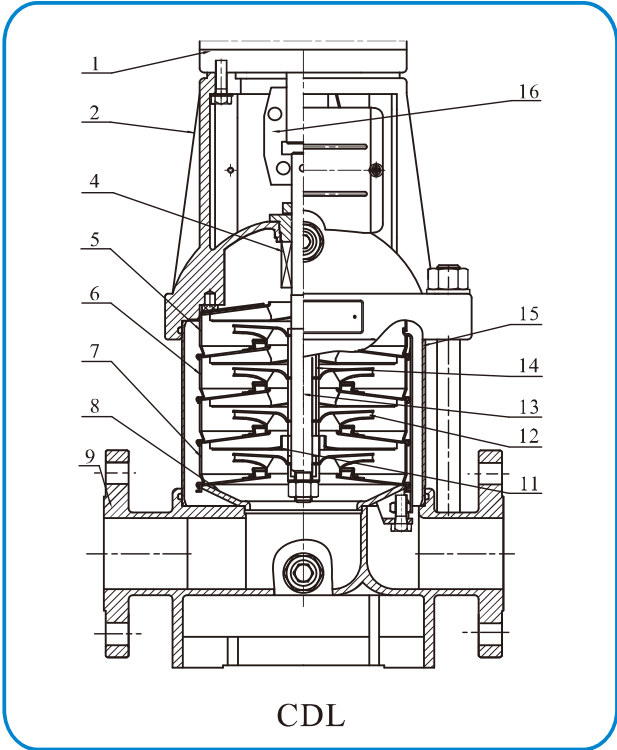
截面图 CDL,CDLF8,10,12,15,20
