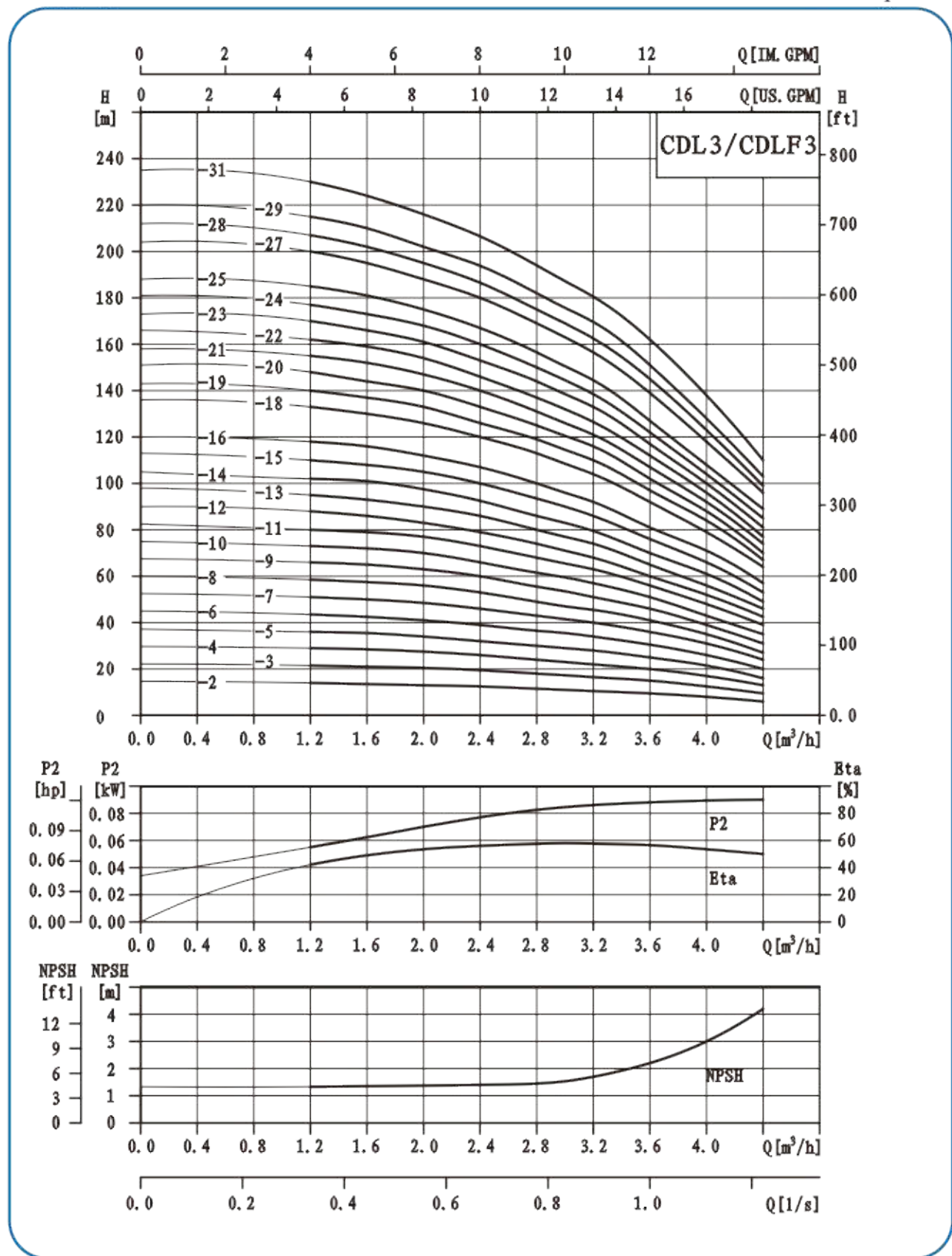
性能曲线
