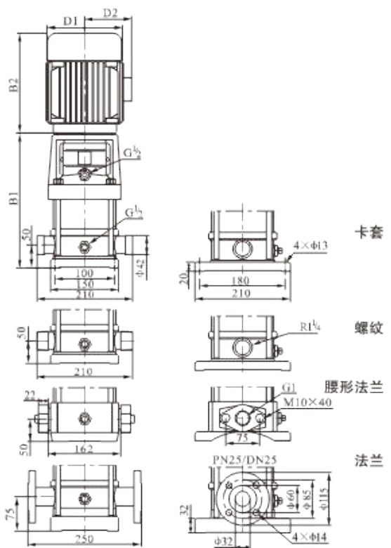
安装图
