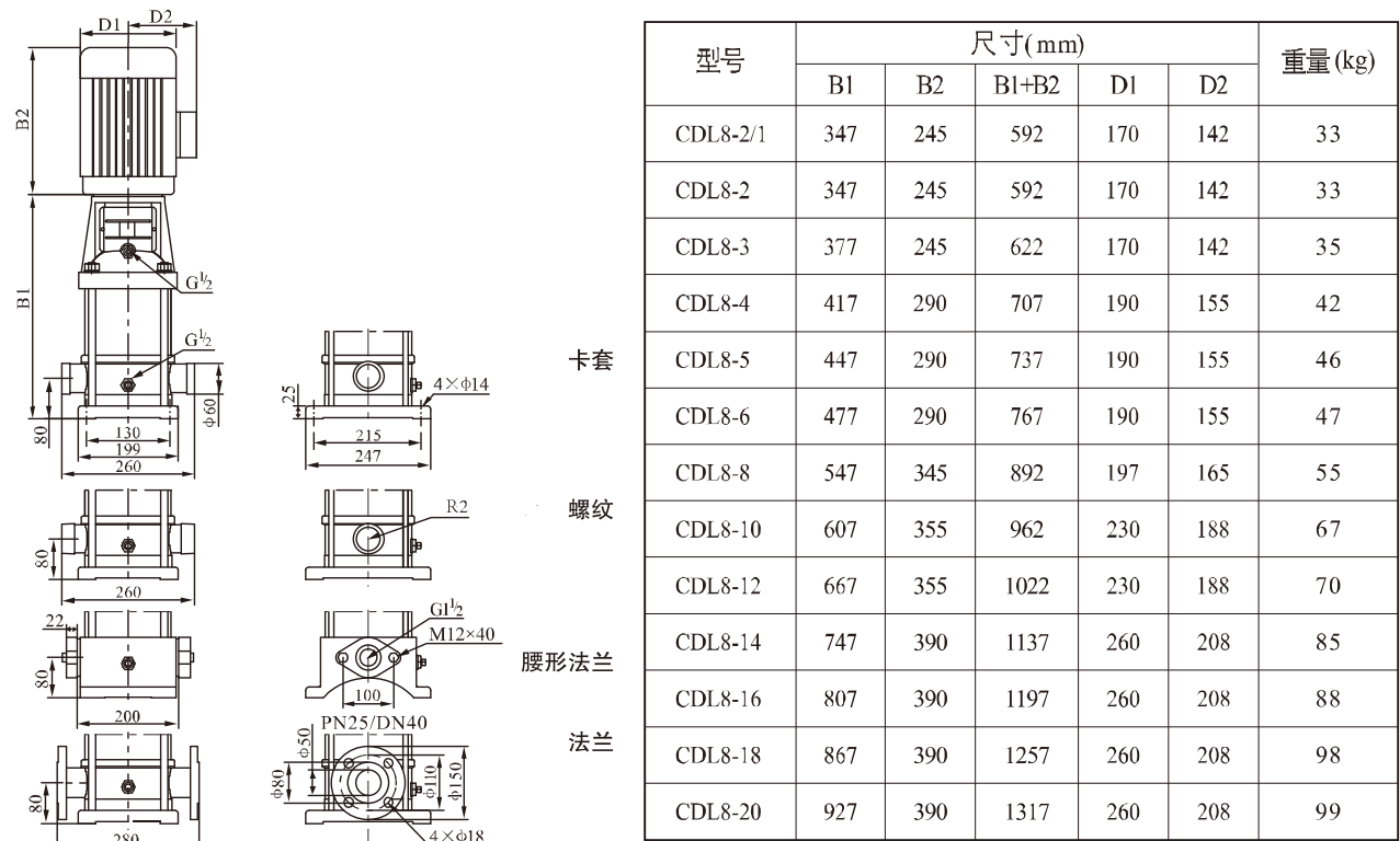
安装图
