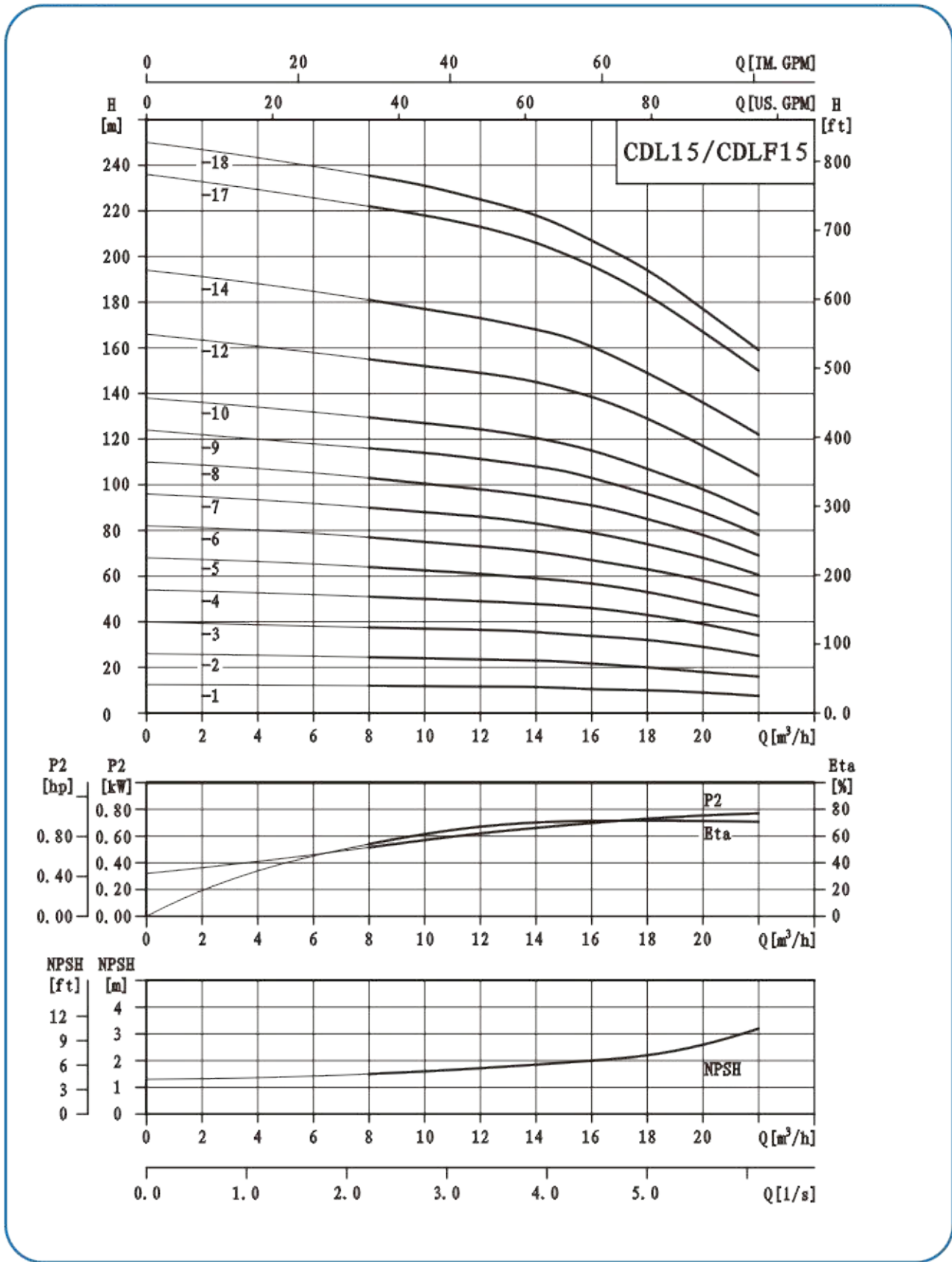
性能曲线
