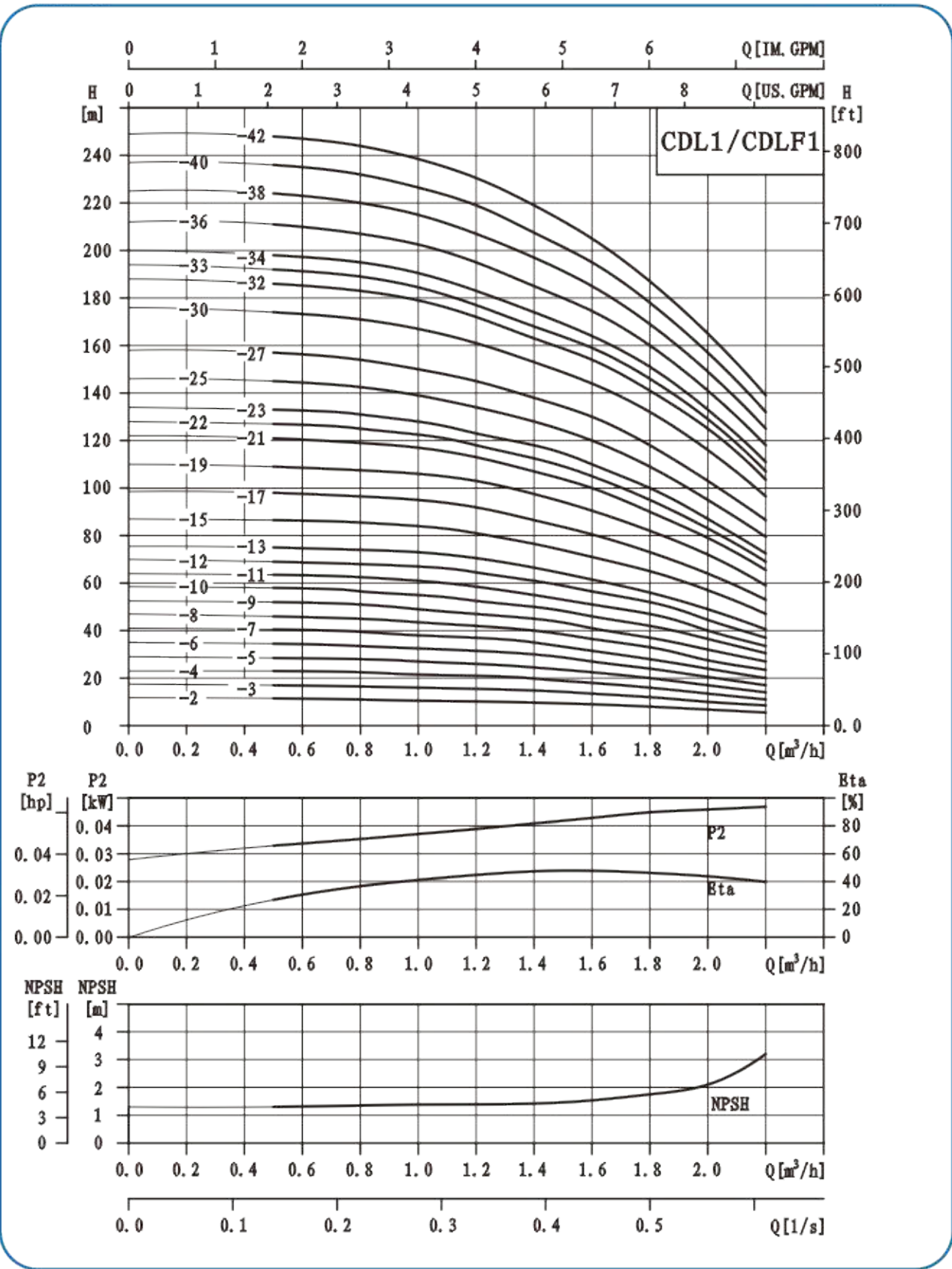
性能曲线
