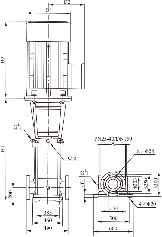
安装图
