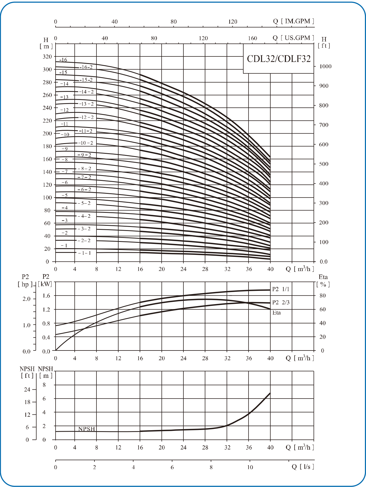
性能曲线 2900rpm
