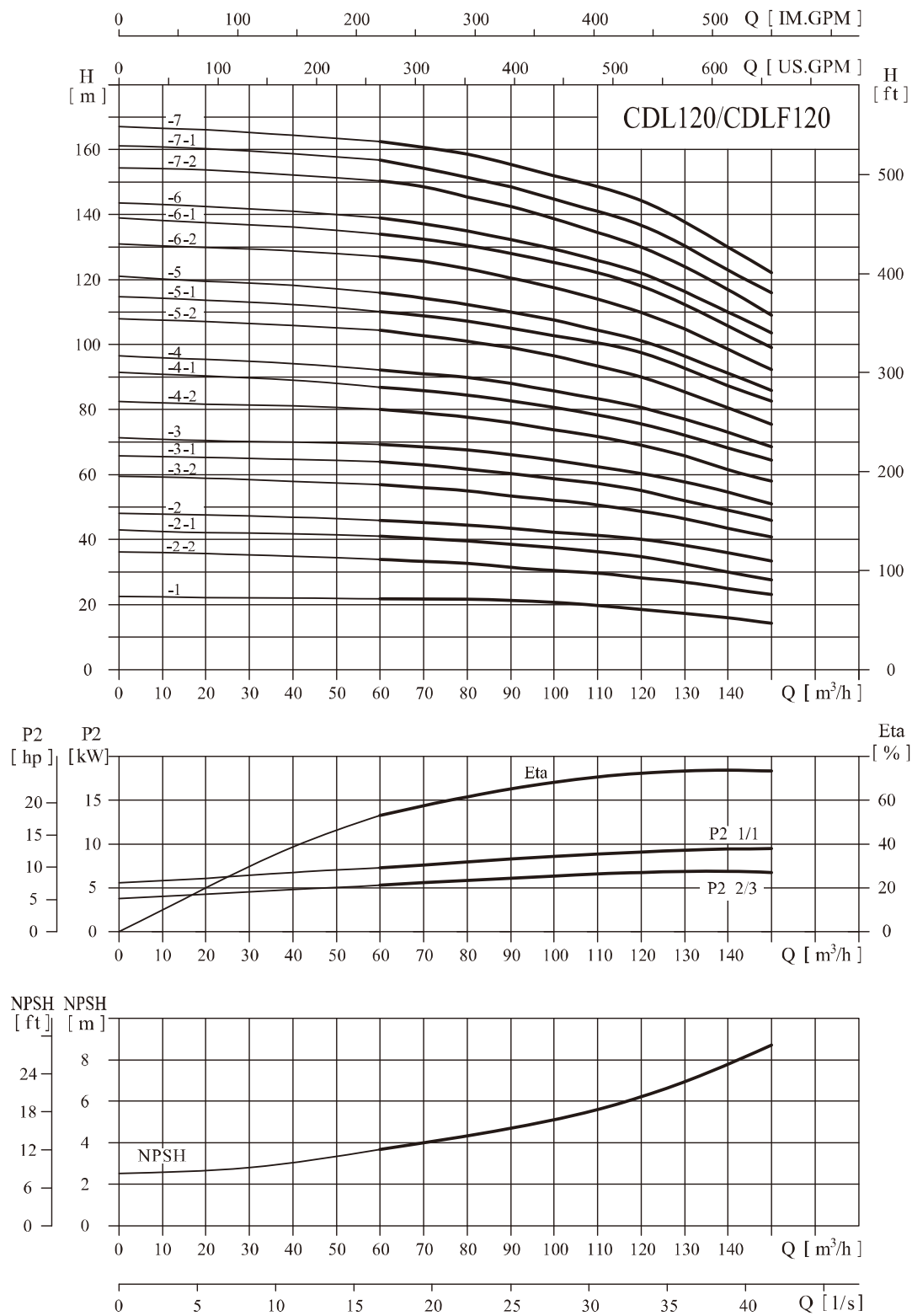
性能曲线
