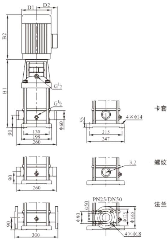
安装图
