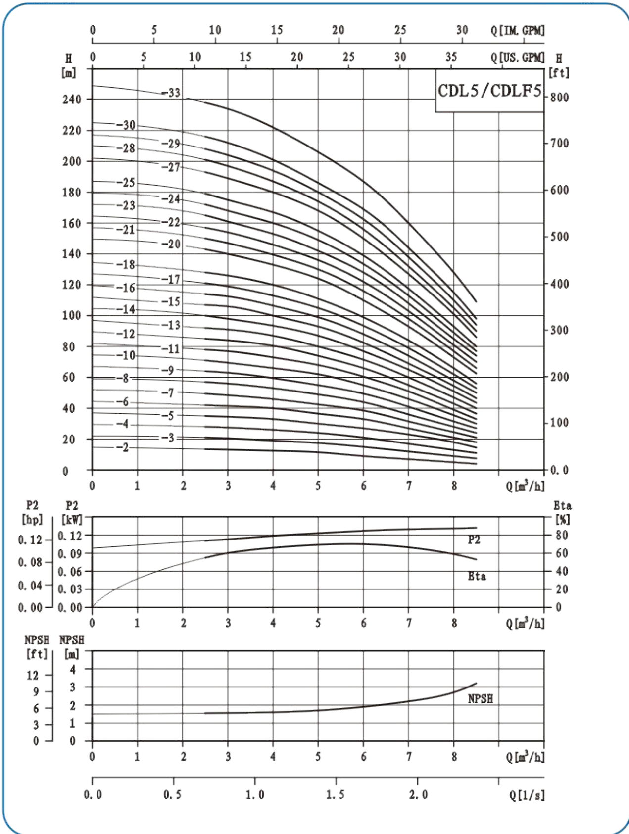
性能曲线
