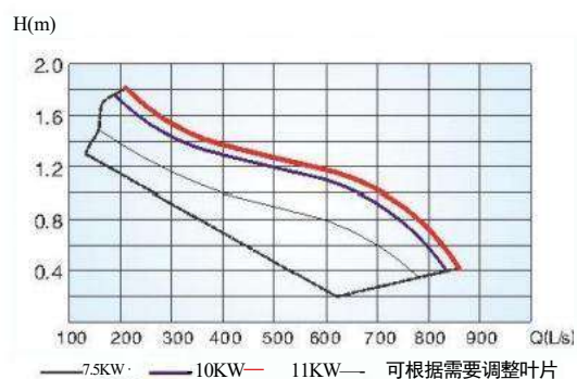
QJB-W7.5
