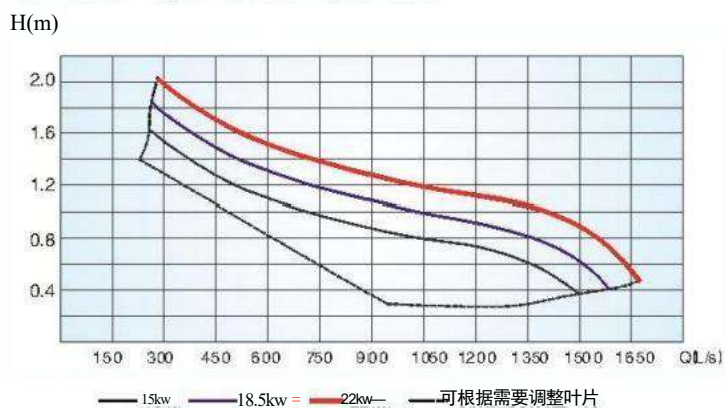
QJB-W15
