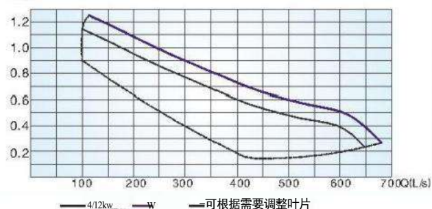
QJB-W4/12 H(m)
