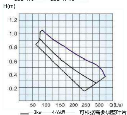
QJB-W3
