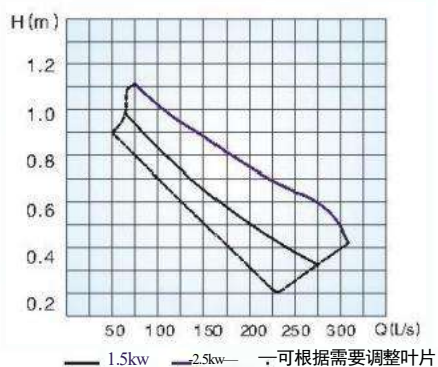
QJB-W4/12 H(m)
