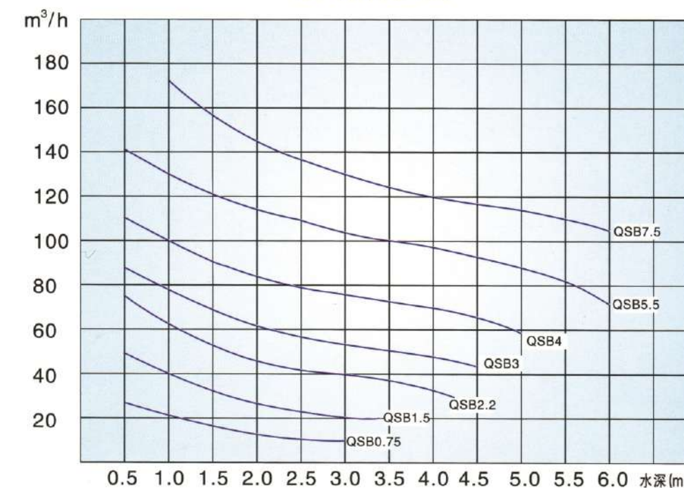
进气特性曲线
