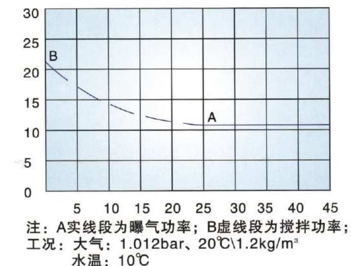
QSB22功能消耗曲线
